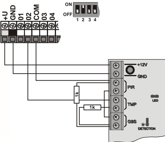
obr. 4 Zapojenie kombinovaného detektora JS-25 Combo do jednej slučky
