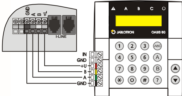
obr. 7 Pripojenie drôtovej klávesnice
