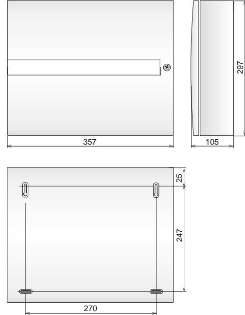
obr. 8 Rozmery skrinky ústredne
