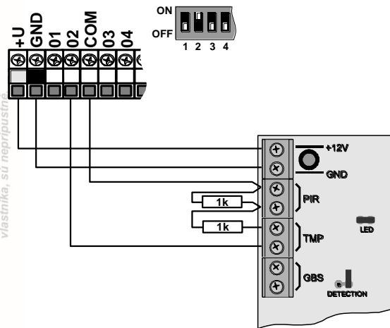
obr. 3 Zapojenie pohybového detektora JS-20 Largo
