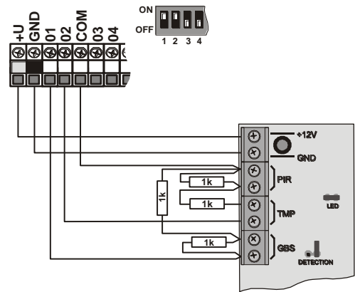
obr. 5 Zapojenie JS-25 Combo do dvoch slučiek (01 GBS, 02 PIR)
