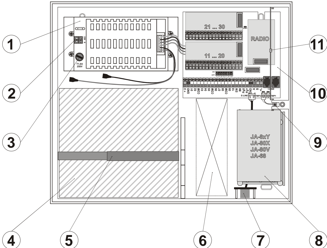
obr. 9 Rozmiestnenie v skrinke ústredne
