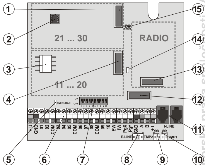
obr. 1 Základná doska (elektronika) ústredne
