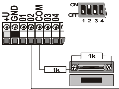
obr. 2 Zapojenie magnetického detektora SA-200
